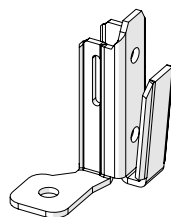
35700902 (5 kpl.) Lattiakiinnikesarja UR, oikea
